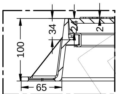
DETALLE B
