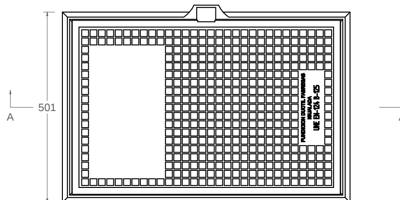
vista en planta 1:10
