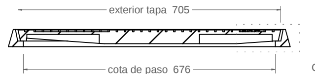
CORTE A-A 1:10
