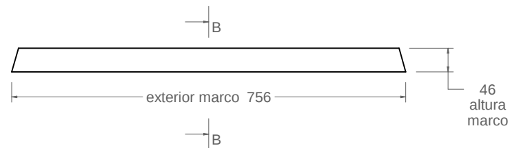
vista alzado 1:10
